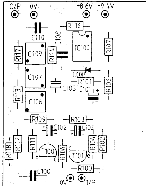
Phono PCB 2225-2-66
